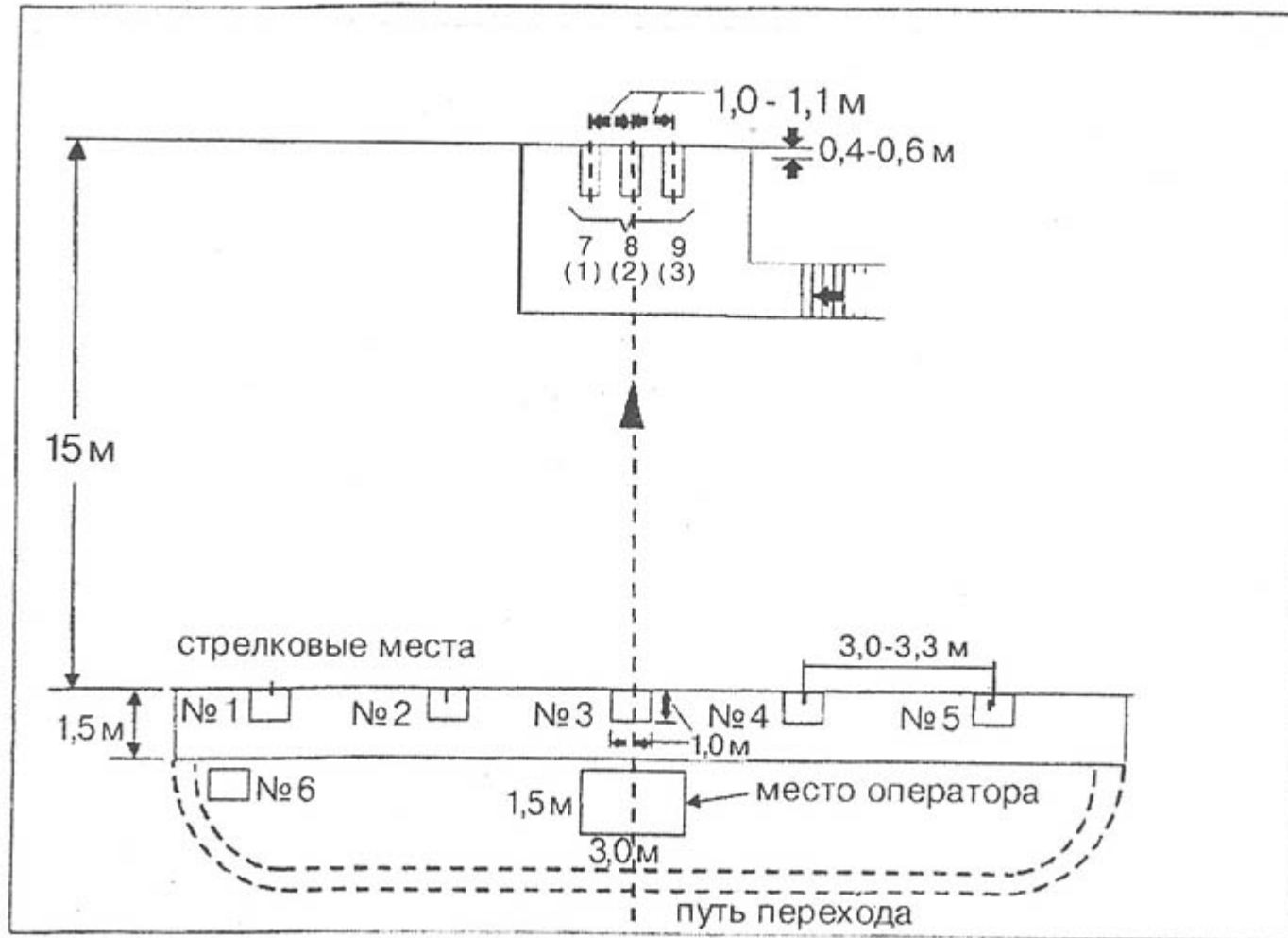
Рисунок 11: Площадка Дубль Трап
