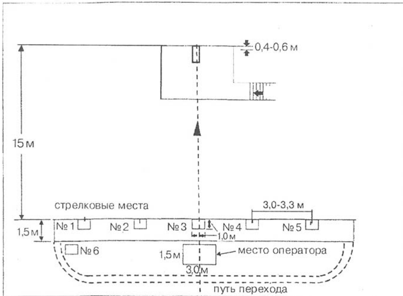
Рисунок 12: Площадка Автоматический Трап
